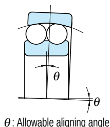
\theta : Allowable aligning angle
